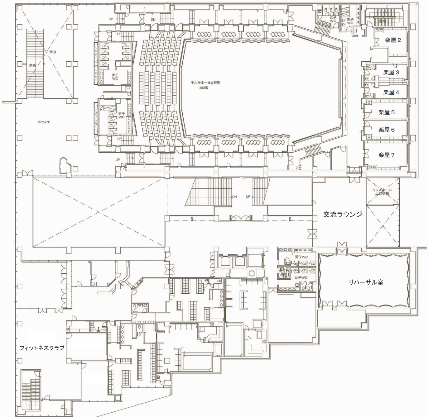
2階 平面図
